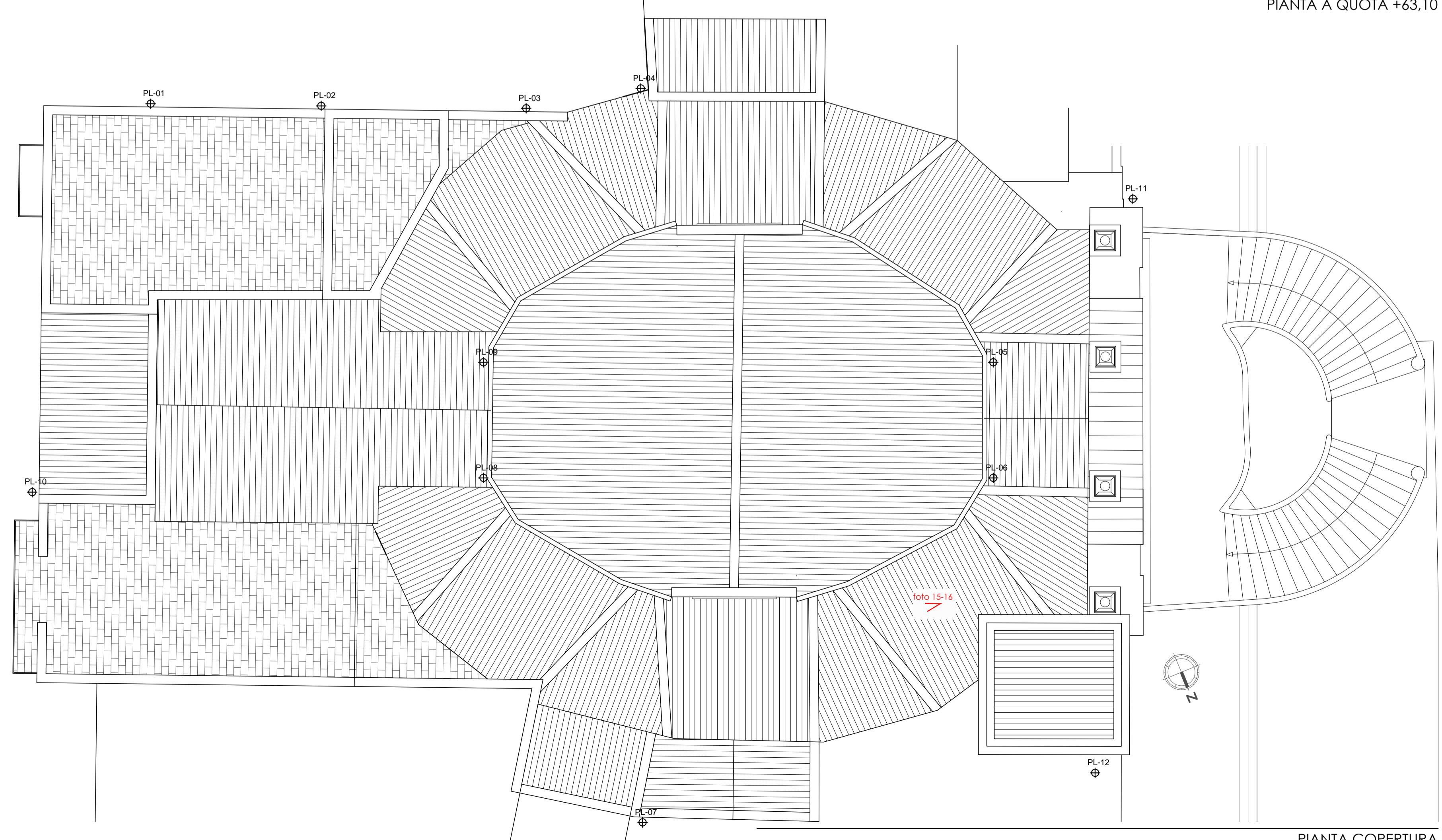
PIANTA COPERTURA
