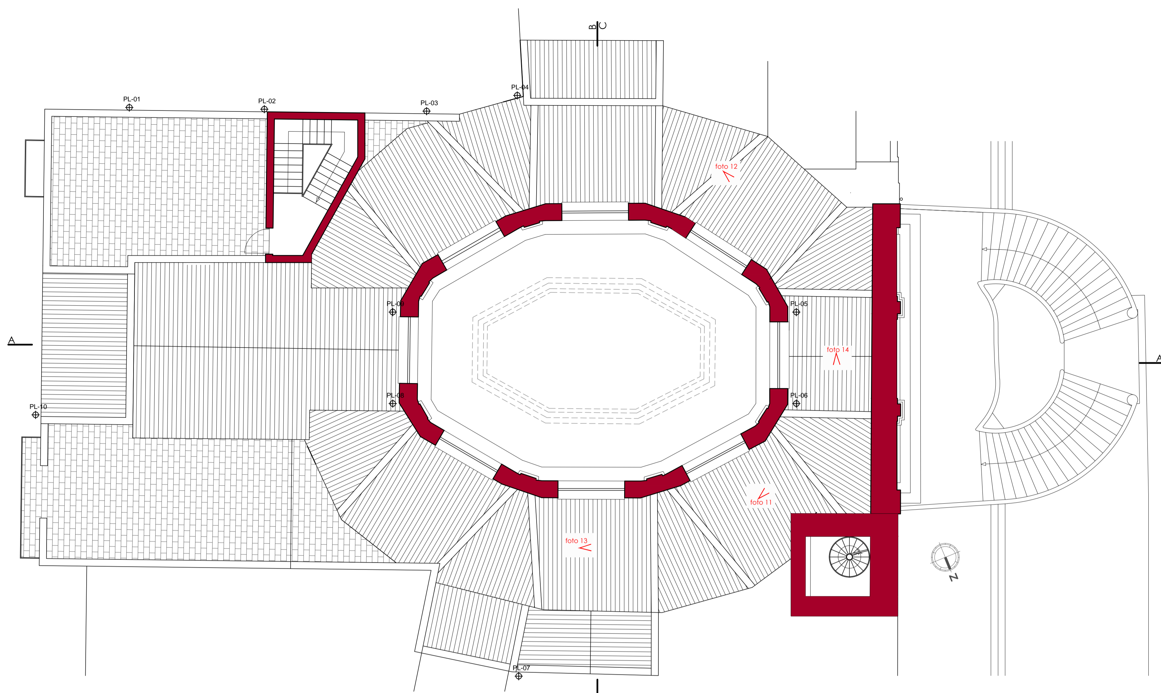
PIANTA A QUOTA +63,10
