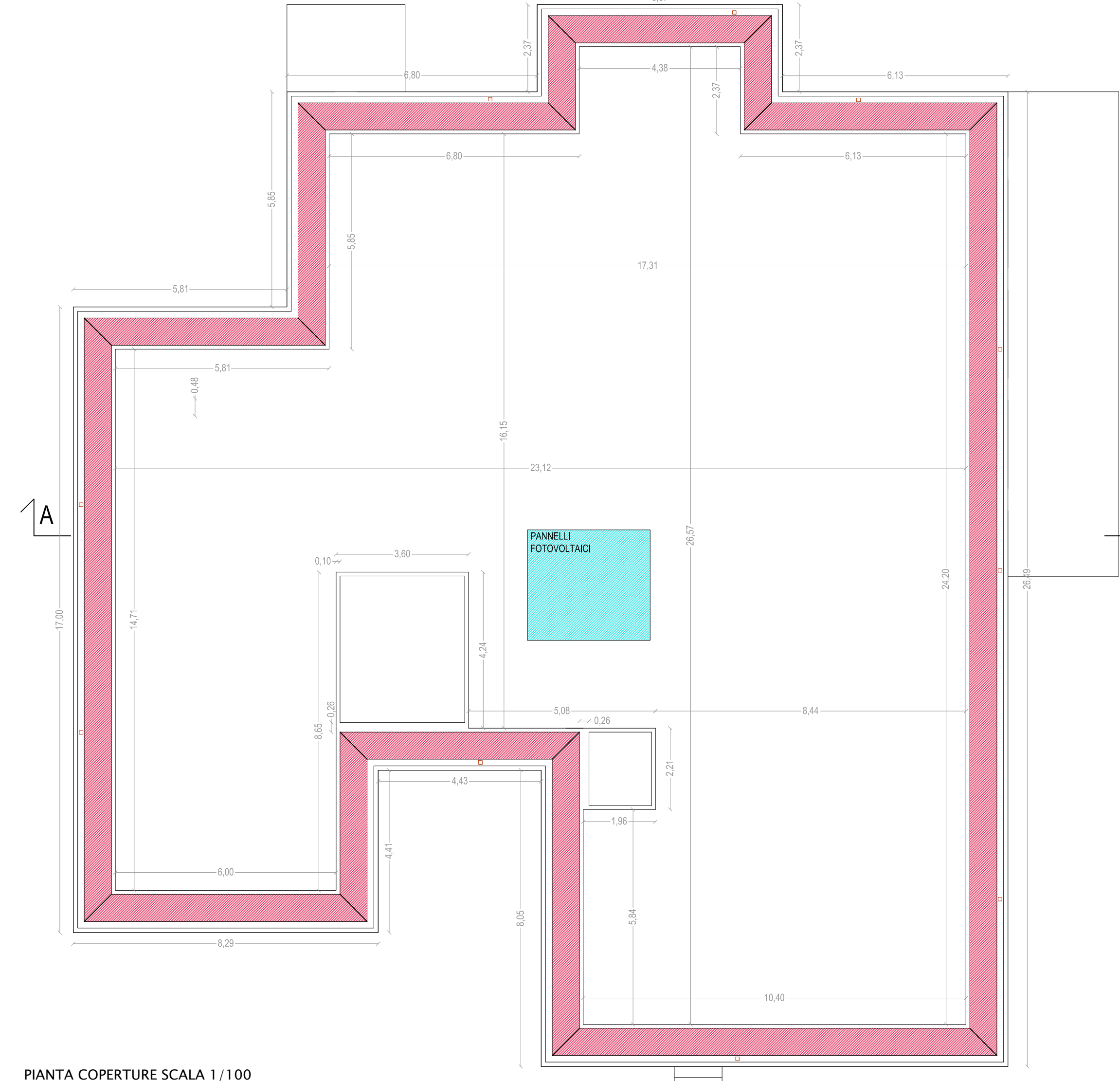
PIANTA COPERTURE SCALA 1/100
